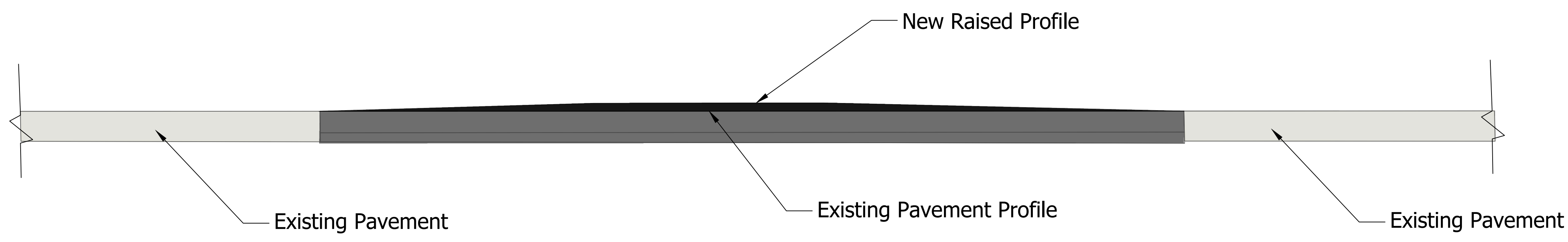
SECTION A-A
